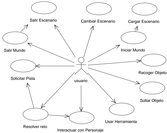
Ilustración 5 - Diagrama de casos de uso para un micromundo interactivo
